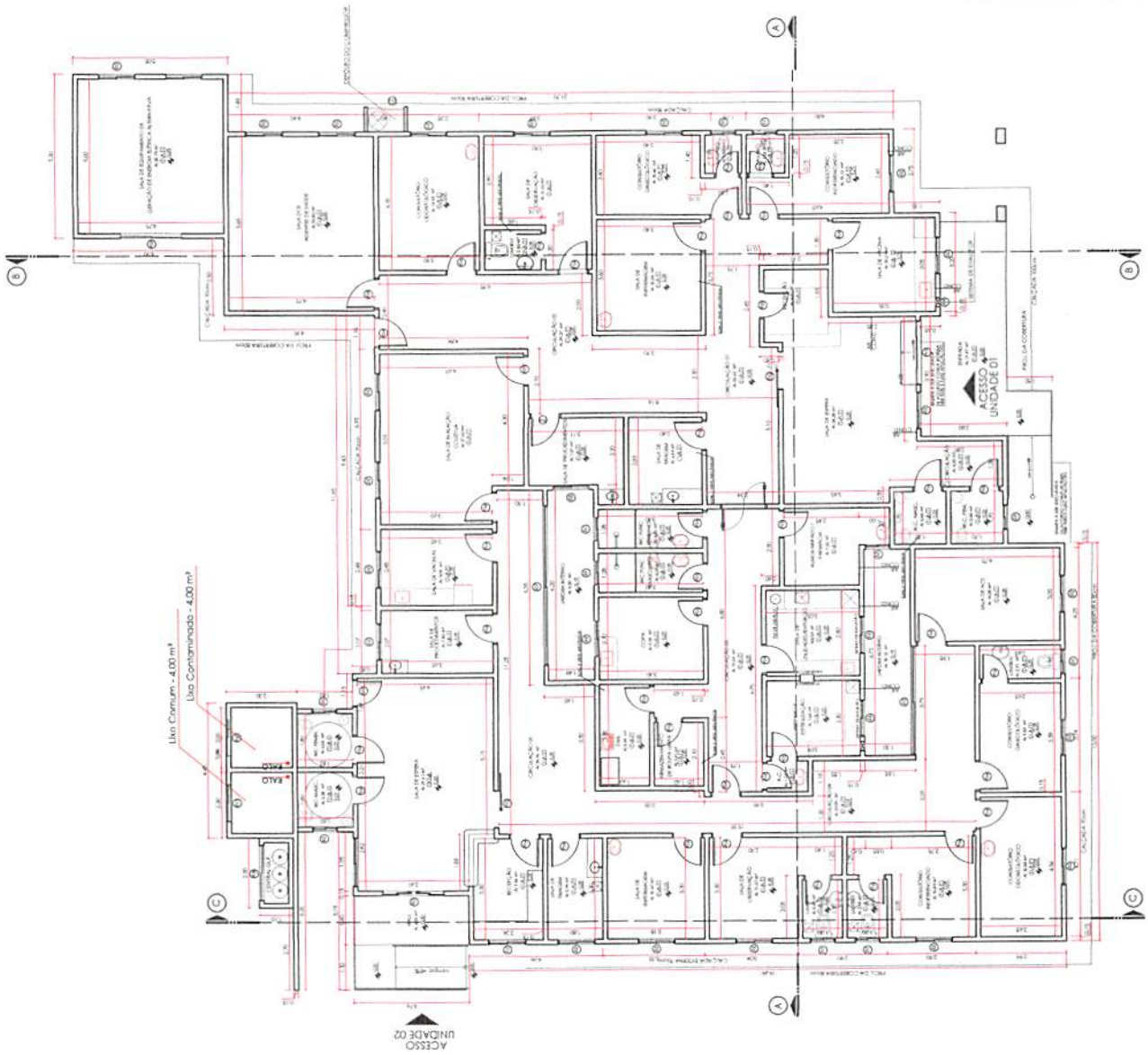
PLANTA BAIXA FINAL Esc: 1/75 Área Externo: 257,01 m² Área a Construir: 362,97 m² ÁREA TOTAL DA EDIFICAÇÃO: 619,98 m²
